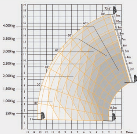
540-180 Stabilisatoren chassis uitgeschoven
