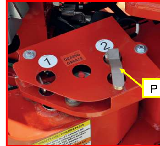
Afbeelding 18: instelling handelingen op stempelpoten.
