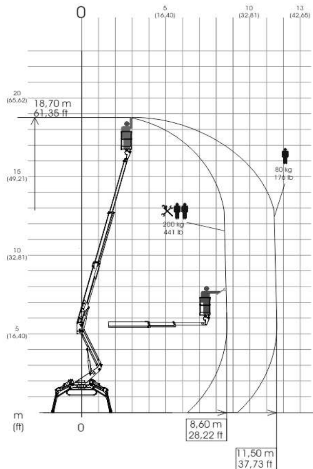
Afbeelding 2a: werkschema.
