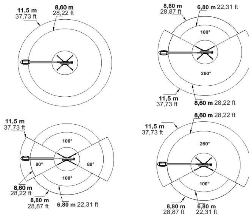
Afbeelding 2b: stabilisatiegebieden.
