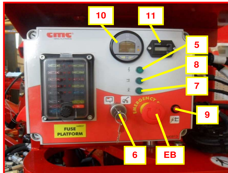
Afbeelding 4b: bedieningspost start/stop motor in geval van hybride versie of full lithium.
