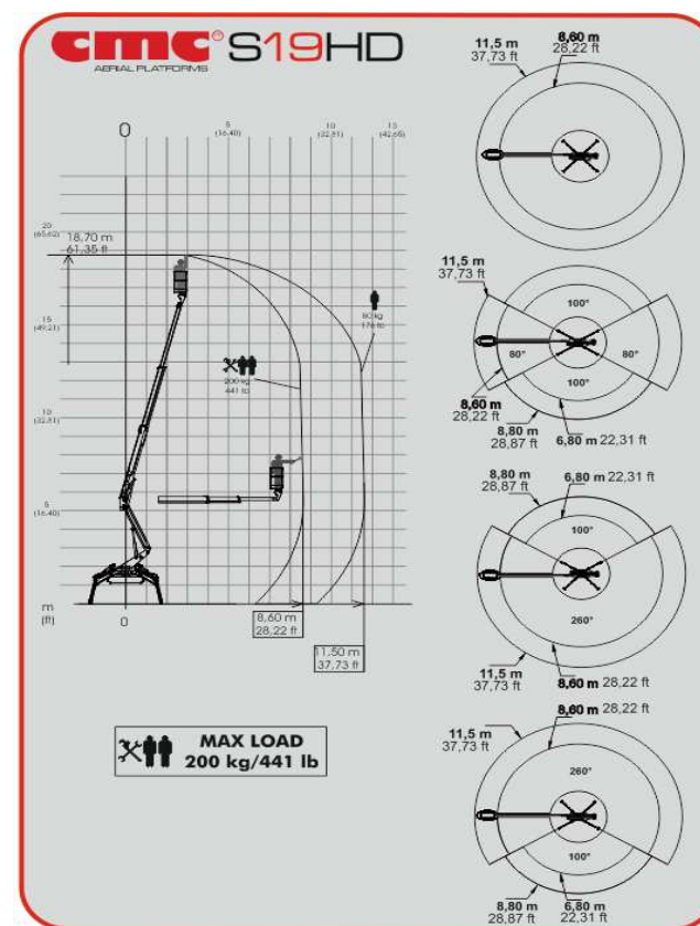
Afbeelding 33: werkschema.
