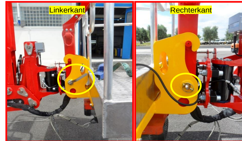
Afbeelding 19: montage korf.
