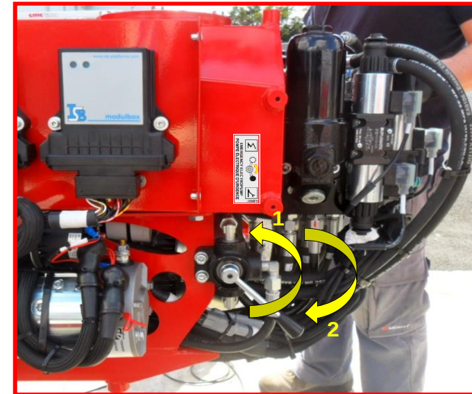
Afbeelding 30: hendel voor gebruik elektrische pomp.
