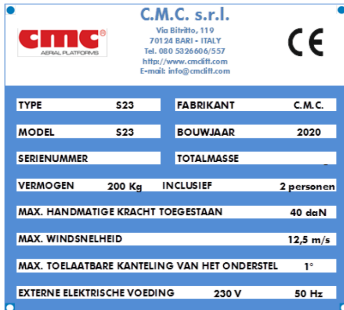
Afbeelding 1: typeplaatje.
