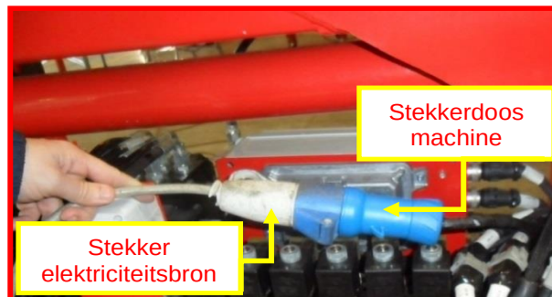
Afbeelding 6: aansluiting 120/230 V-stekker.
