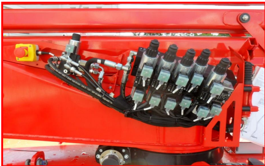
Afbeelding 15: kleppengroep noodbedieningspost.
