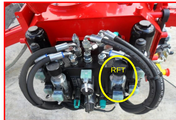
Afbeelding 26: klep rechts van de filtergroep.
