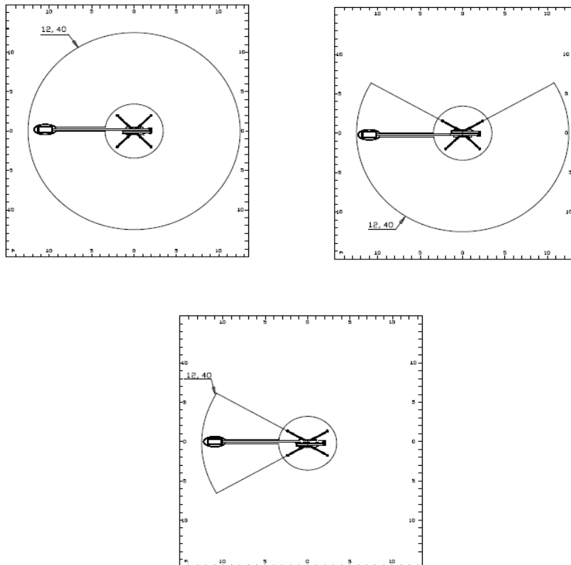
Afbeelding 2b: werkgebied.
