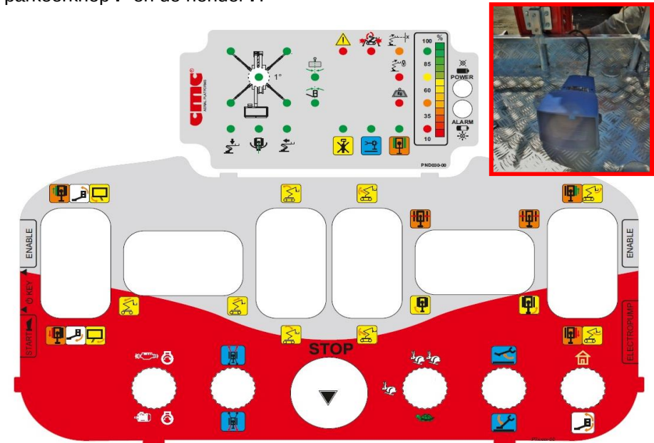
Afbeelding 12: bedieningspost in de korf + “dodemenspedaal”.
