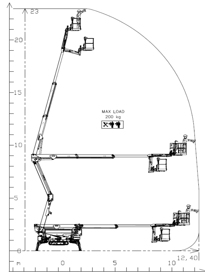
Afbeelding 2a: werkschema.
