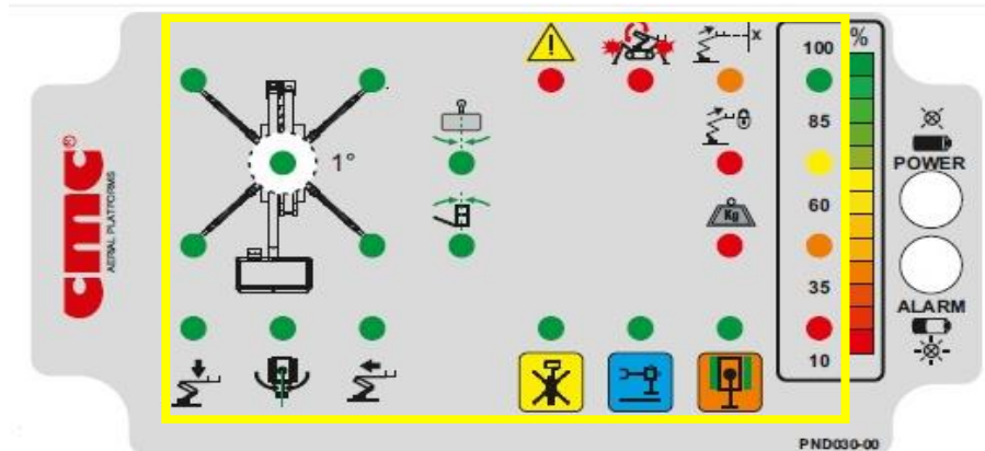
Afbeelding 9: LED-paneel met waarschuwinglampjes.
