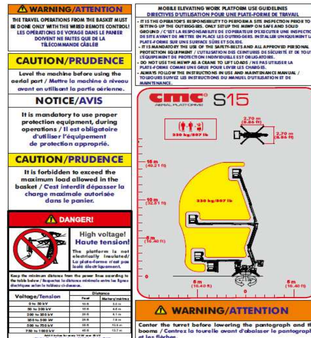
Figure 31 : indications dans le panier.
