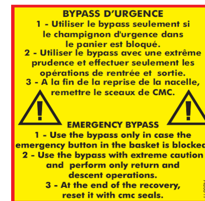
Figure 61 : indications pour utilisation du by-pass d'urgence.
