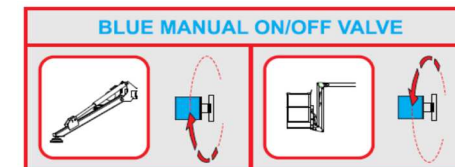
Figure 19 vanne bleue pour échange d'alimentation stabilisateurs/partie aérienne.
