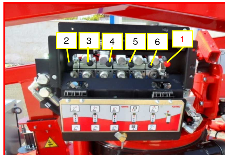
Figure 11 : poste de commande (de secours) plateforme.
