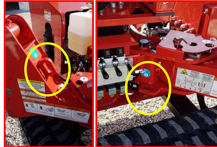
Figure 16 : crochets sur le châssis pour élinguer la PEMP.
