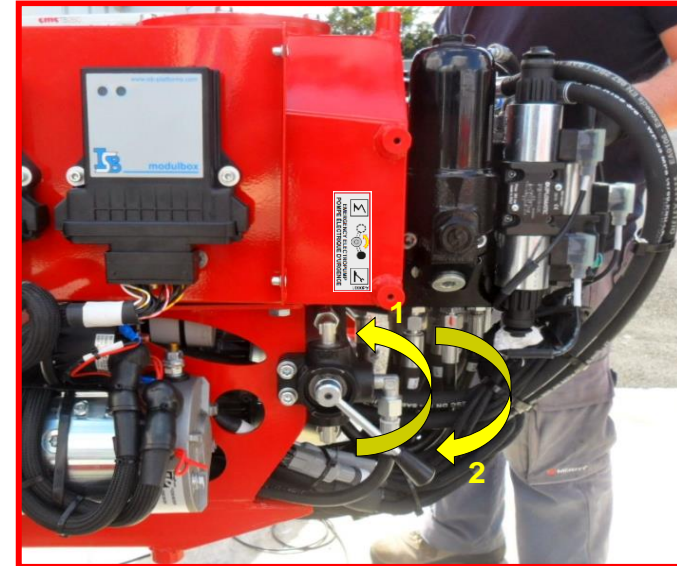
Figure 30 : robinet utilisation de l'électropompe.
