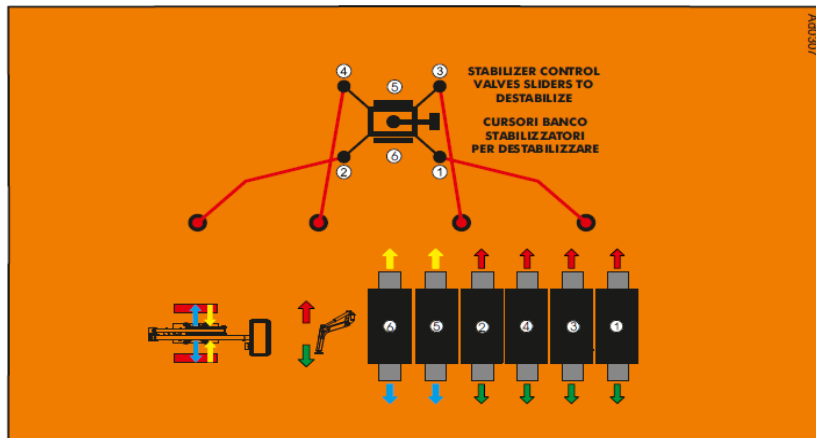
Afbeelding 101: manoeuvres voor destabilisatie op bedieningspaneel stempelpoten.
