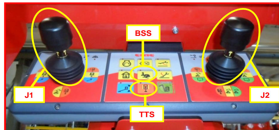
Figure 23 : poste de commande translation (dans nacelle).
