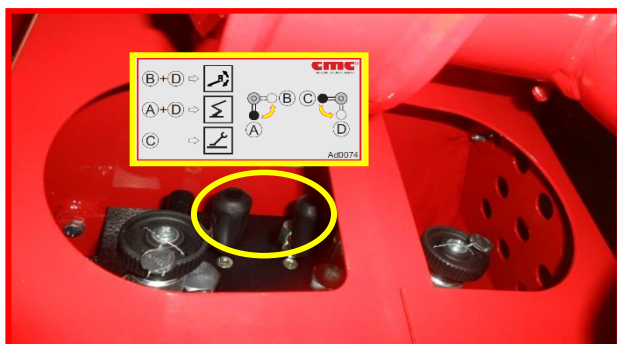
Figure 40 : robinet pour utilisation de la pompe manuelle.
