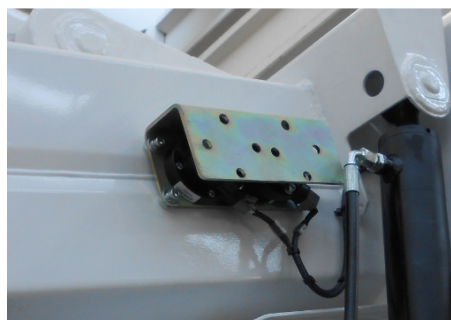
fig. 2.10.6 Transducteurs d'angle télescopiques
