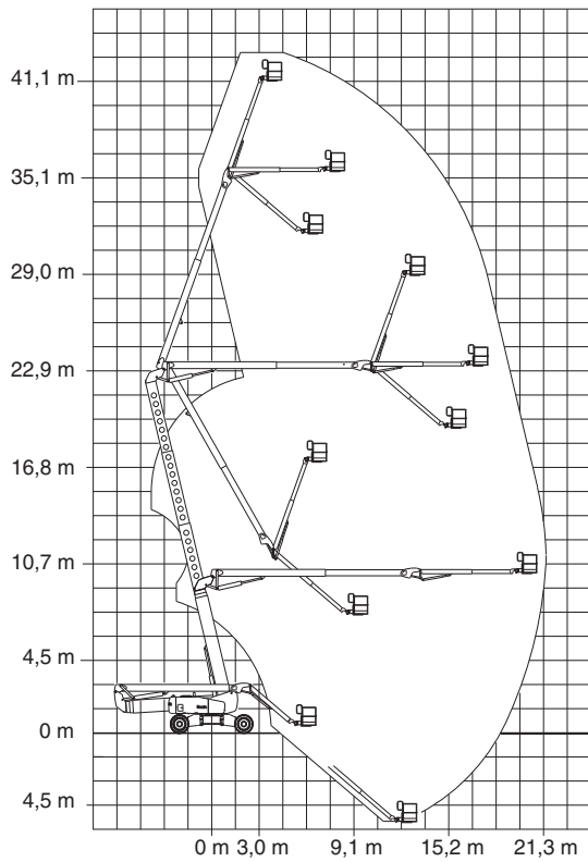
Diagram werkbereik ZX-135/70
