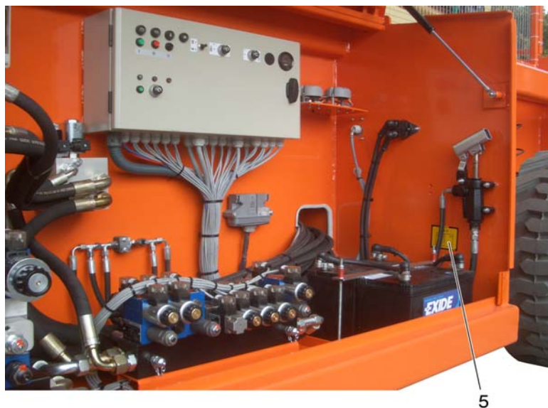
Compartiment des soupapes et compartiment électrique
