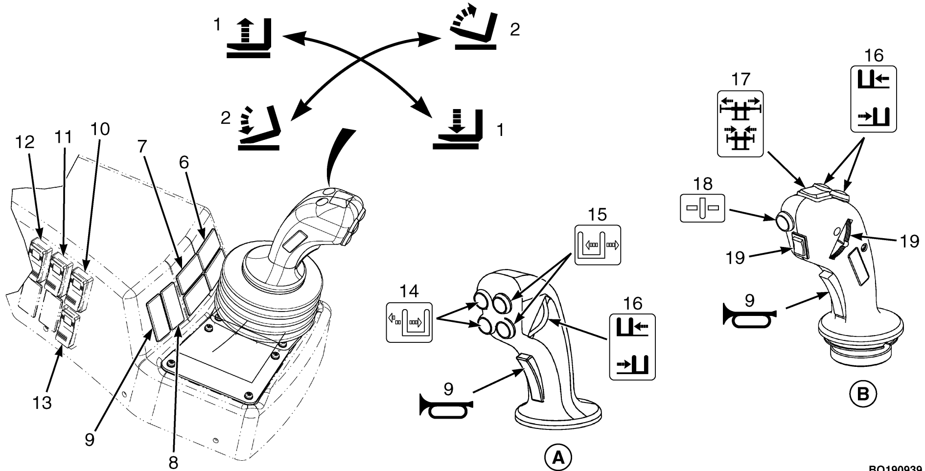
Figure 11. Commandes et interrupteurs de l'accoudeoir (joystick en option) (Elément 2 de 2)
