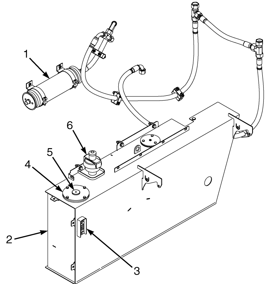
Figure 22. Eléments d'entretien de réservoir hydraulique
