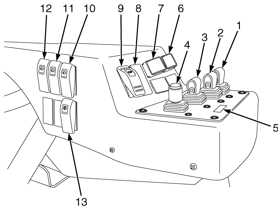
Figure 10. Commandes et interrupteurs de l'accoudoir (joystick en option) (Elément 1 de 2)
