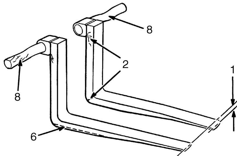
Figure 16. Vérification de l'état des fourches
