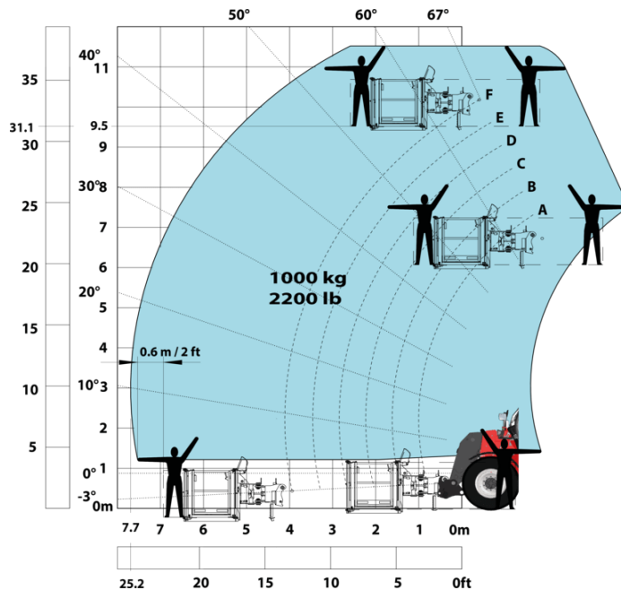
Machine sur pneus avec nacelle Métric
