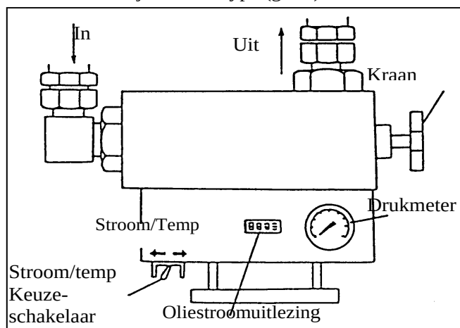
Typische oliestroommeter uitgerust met smoorventiel
