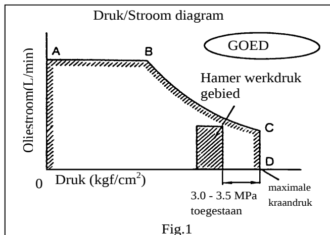
Voorbeeld van Druk/Stroom curve
