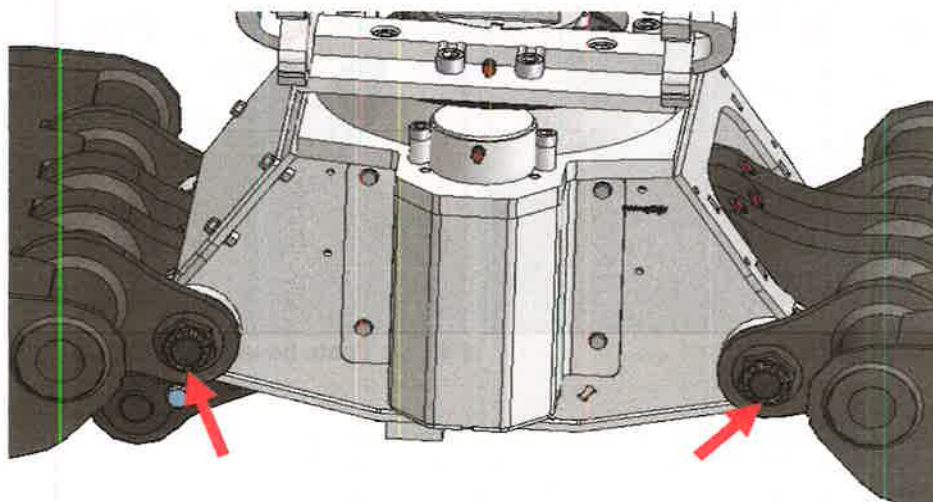
Fig. 15: Kroonmoeren met spanbusborging
