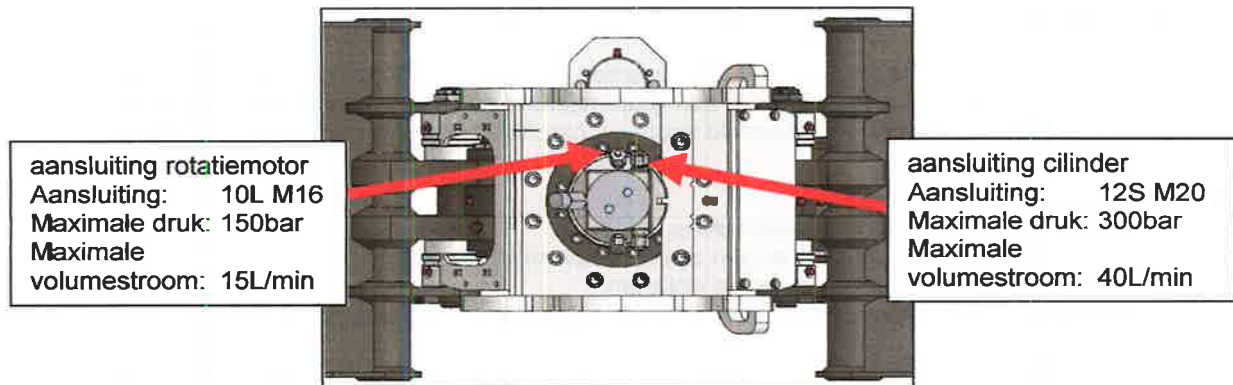
Fig. 8: Hydrauliek-aansluitingen
