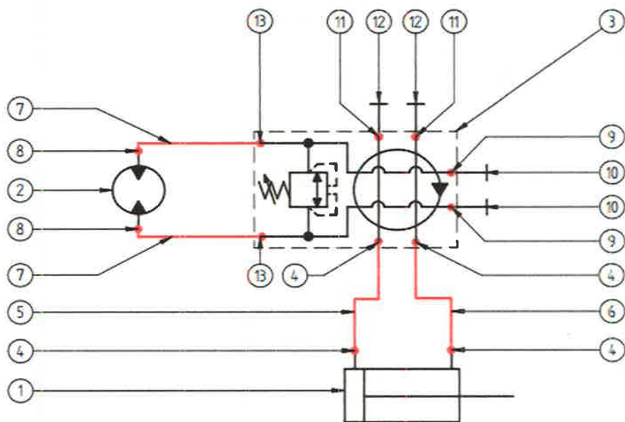
Roteerbare grijper
