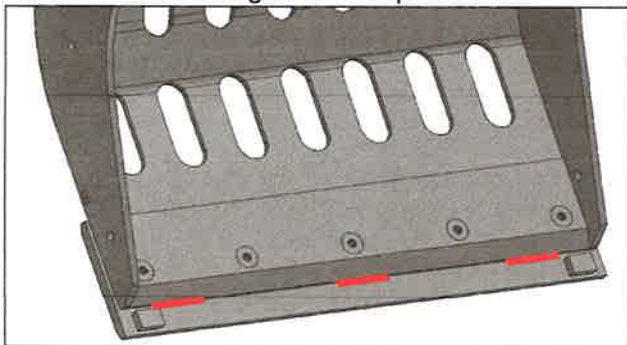
Fig. 14 Positie hechtlassen
