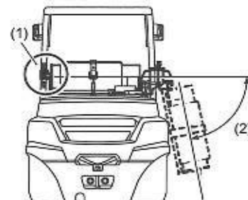
(1) Butée du support du réservoir (2) 65°
