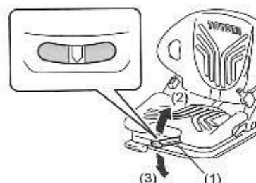
(1) Levier de réglage d'inclinaison du dossier
