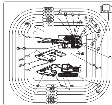
46 Schéma de graissage et d'entretien. Voir page 279.
