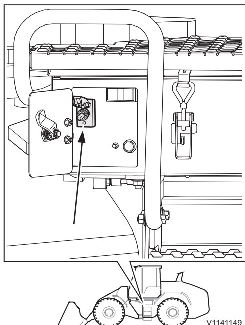
Hoofdstroomschakelaar
