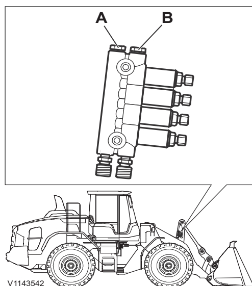
Principeschets
