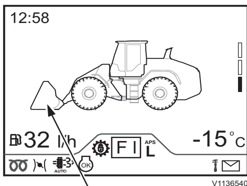
Bedieningsinformatiescherm 3 (alle functies hier weergegeven)
