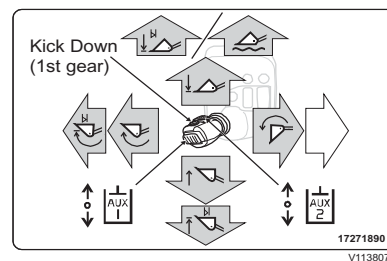
32 Functies voor enkelvoudige hendelbediening
