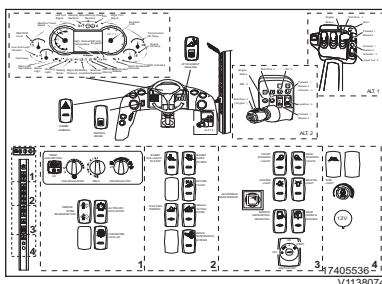
31 Overzicht bedieningselementen in cabine (in het Engels)
